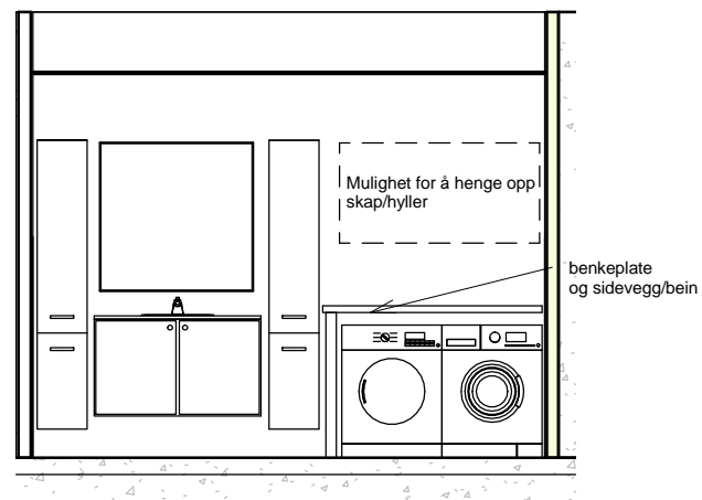
B2 - Bad og vask 1 : 50
